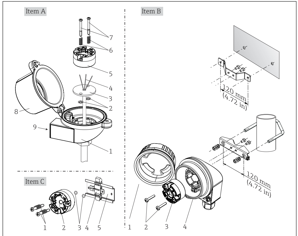
图 1 模块化变送器的安装示意图（三种安装方式）
