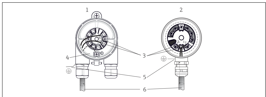
图 6 连接信号电缆和电源
