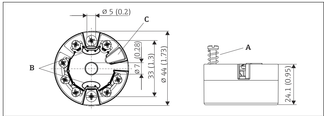
图 18 带螺纹式接线端子的设备型号
