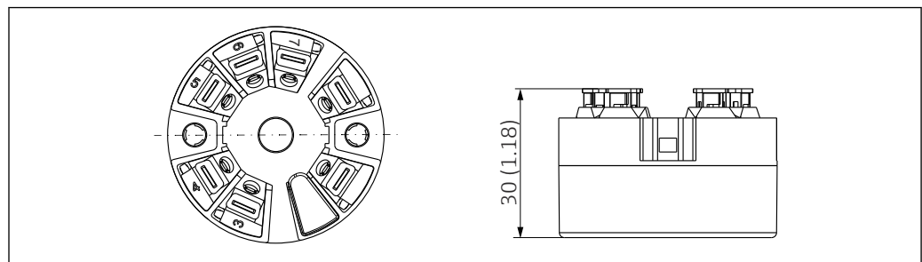
图 19 带直推式接线端子的设备型号。除了外壳高度之外, 其他外形尺寸均与带螺纹式接线端子的设备相同。
