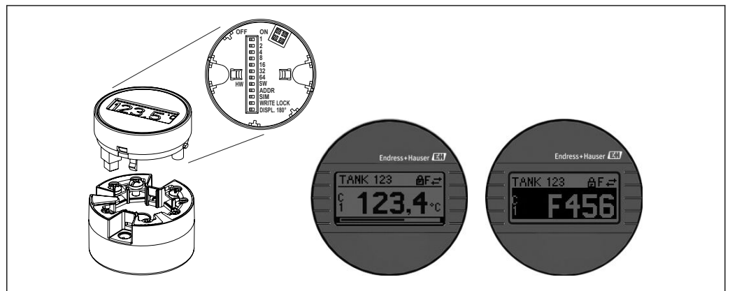
图 20 TID10 插拔式测量值显示单元，带棒图显示（可选）
