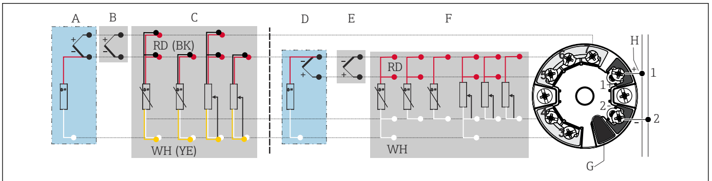
图 5 模块化温度变送器的接线端子分配
