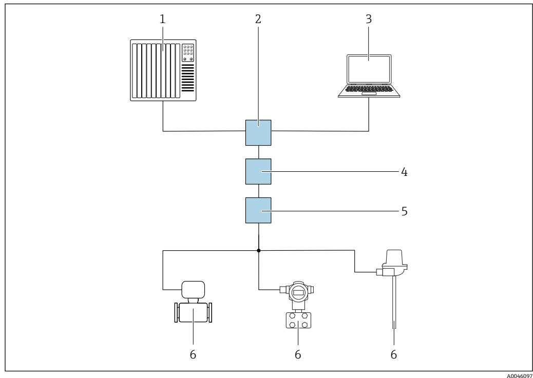
图 11 通过 PROFINET + Ethernet-APL 网络实现远程操作：星形拓扑结构
