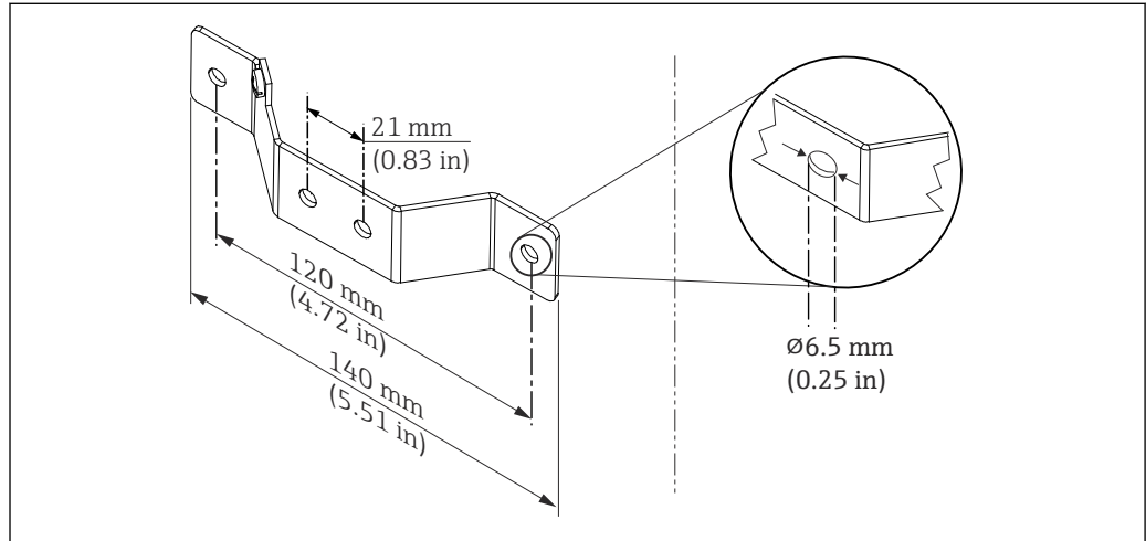
图 2 墙装架的外形尺寸 (整套墙装套件可以作为附件订购)
