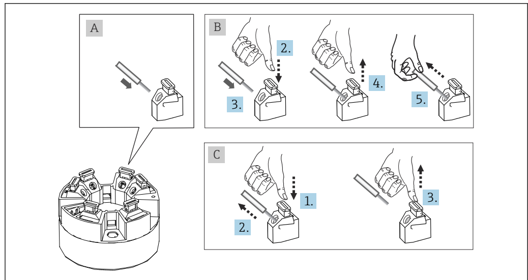
图 7 连接至直推式接线端子
