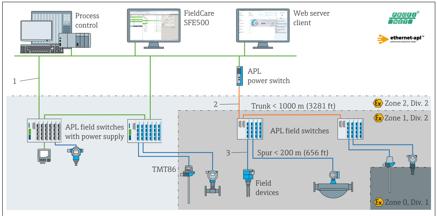
图 17 PROFINET + Ethernet-APL 通信变送器的设备结构示意图
