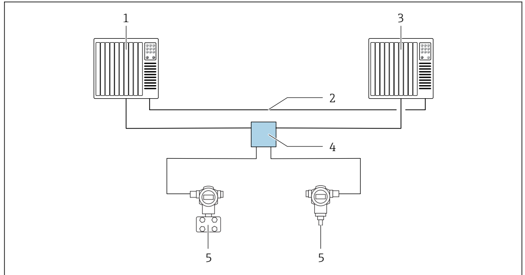
图 13 S2 系统冗余布局实例：星形拓扑结构
