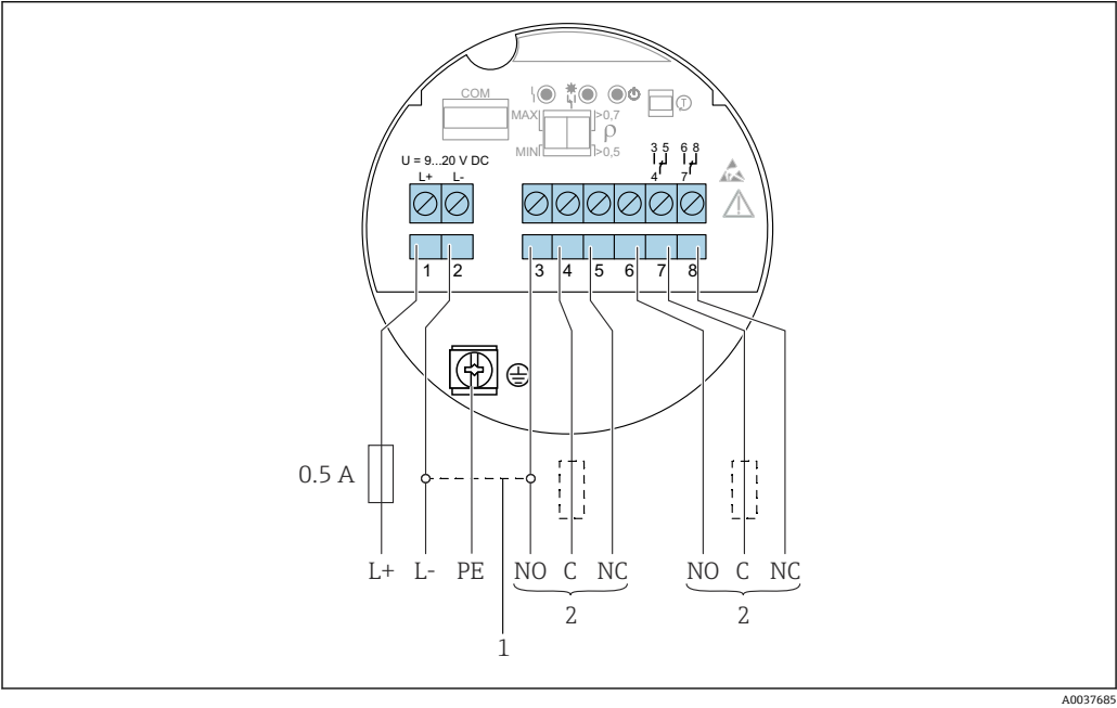
图 23 电子插件 FEL64 DC: 直流连接型，带继电器输出
