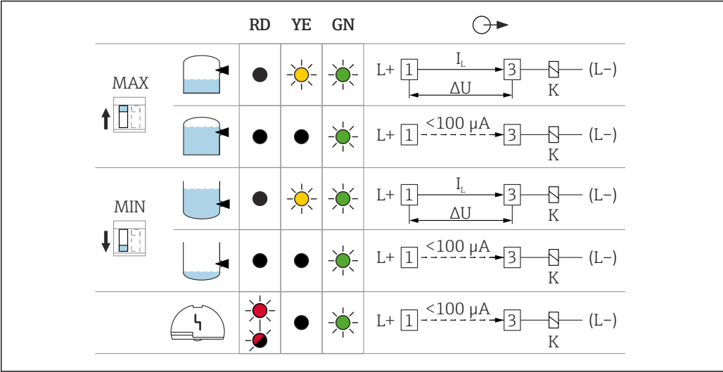
图 20 电子插件 FEL62 的继电器响应和故障信号
