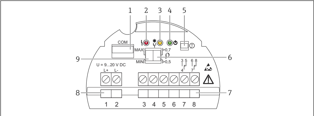
图 32 实例：电子插件 FEL64DC 1 通信接口，用于连接附加模块（LED 指示灯、蓝牙模块） 2 红色 LED 指示灯：警告或报警 3 黄色 LED 指示灯：继电器的开关状态 4 绿色 LED 指示灯：工作状态（设备开启） 5 测试按钮，用于执行功能测试 6 DIP 开关，密度设定值为 0.7 或 0.5 7 继电器触点接线端子（3...8） 8 电源接线端子（1...2） 9 DIP 开关，高限（MAX）/低限（MIN）检测设置
