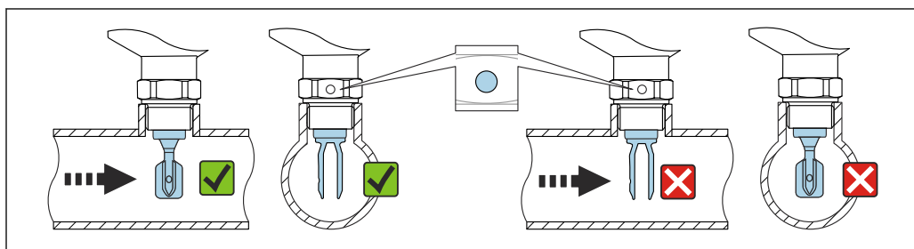
图 12 安装在管道中（考虑叉体安装位置和标记）
