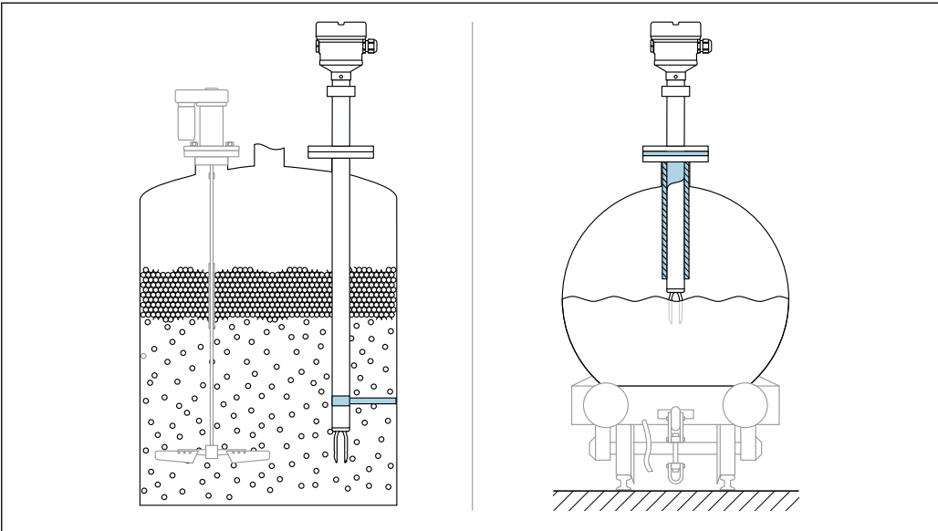
10 存在动态负载时，支撑设备的实例
