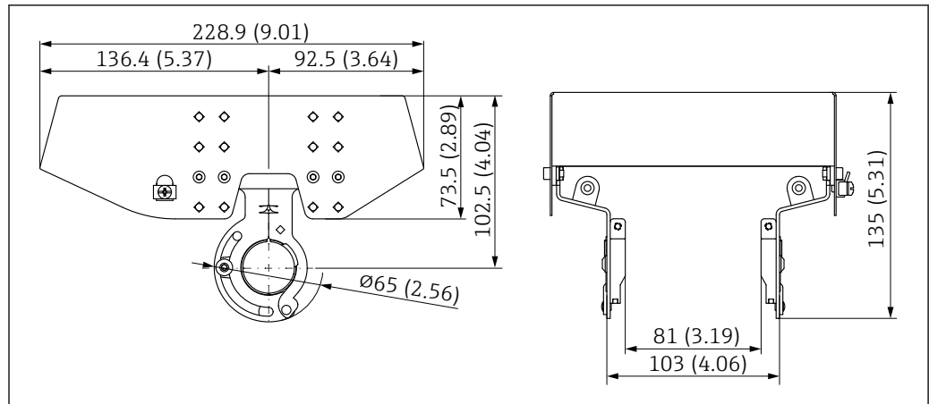
图 44 防护罩，适用双腔室铝外壳。测量单位 mm (in)
