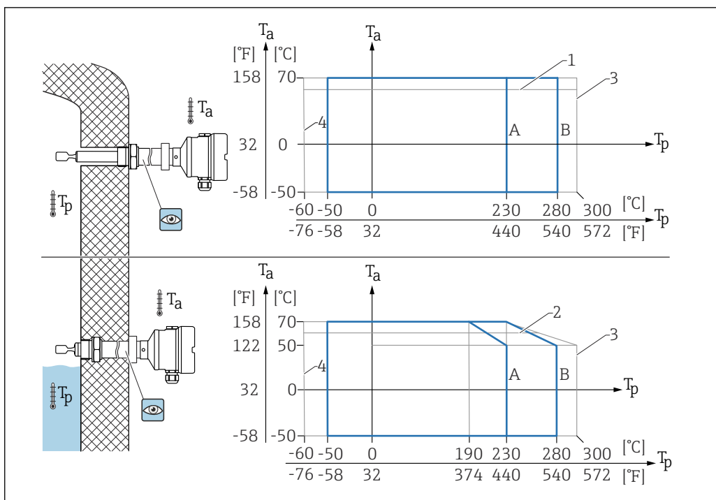
图 52 外壳允许环境温度 T_a 与罐体内部过程温度 T_p 的关系
