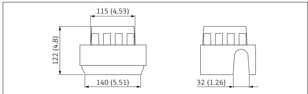
图 45 保护盖，适用单腔室铝外壳或 316L 外壳。测量单位 mm (in)
