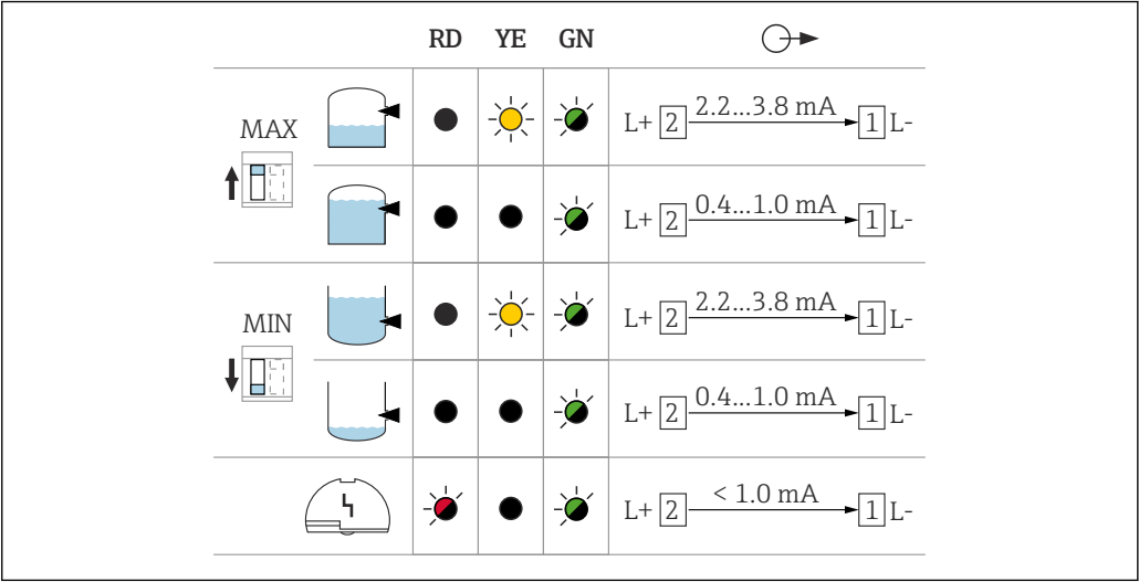
28 电子插件 FEL68 的开关量输出和信号传输
