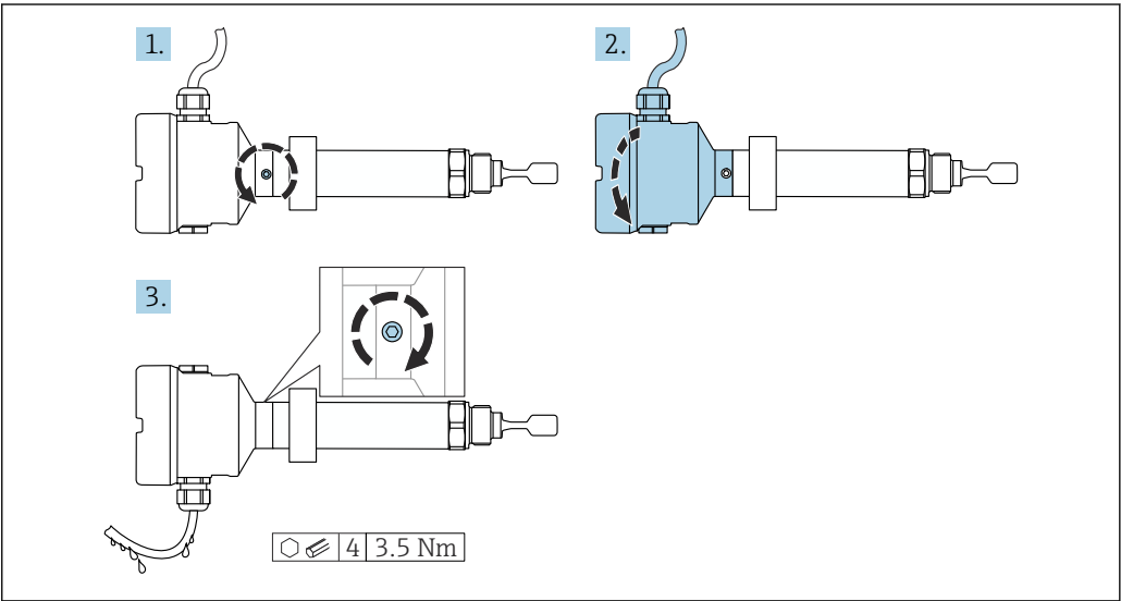
14 外壳带外部锁定螺丝和排水回路
