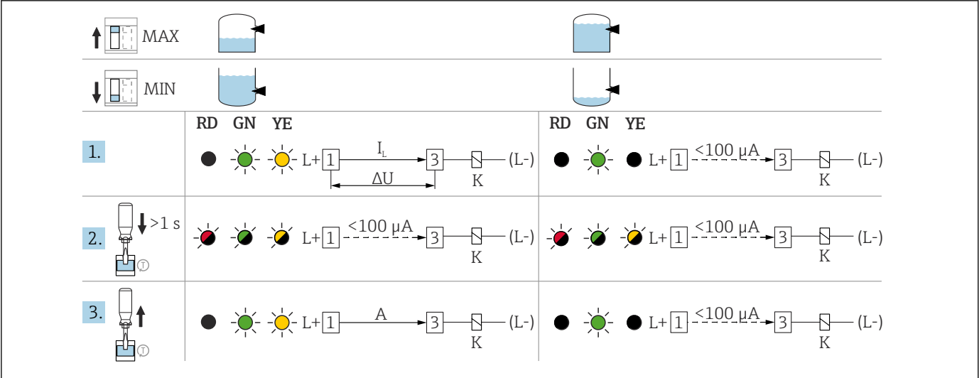
36 FEL62 的继电器响应和故障报警信号
