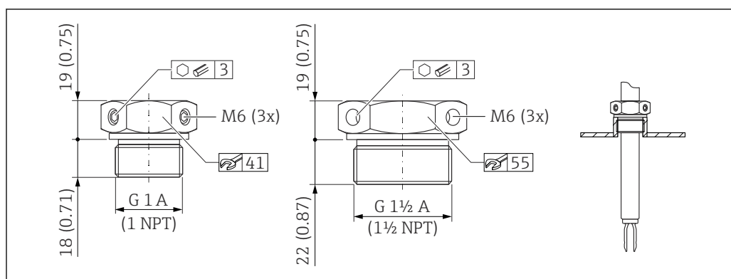
图 50 常压活动套管 p_e = 0 \text{ bar} (0 psi)。测量单位 mm (in)
