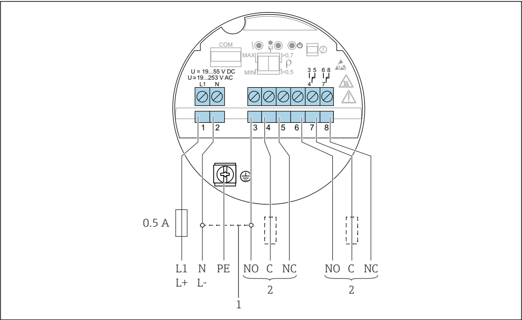
21 电子插件 FEL64：通用电流连接型，带继电器输出
