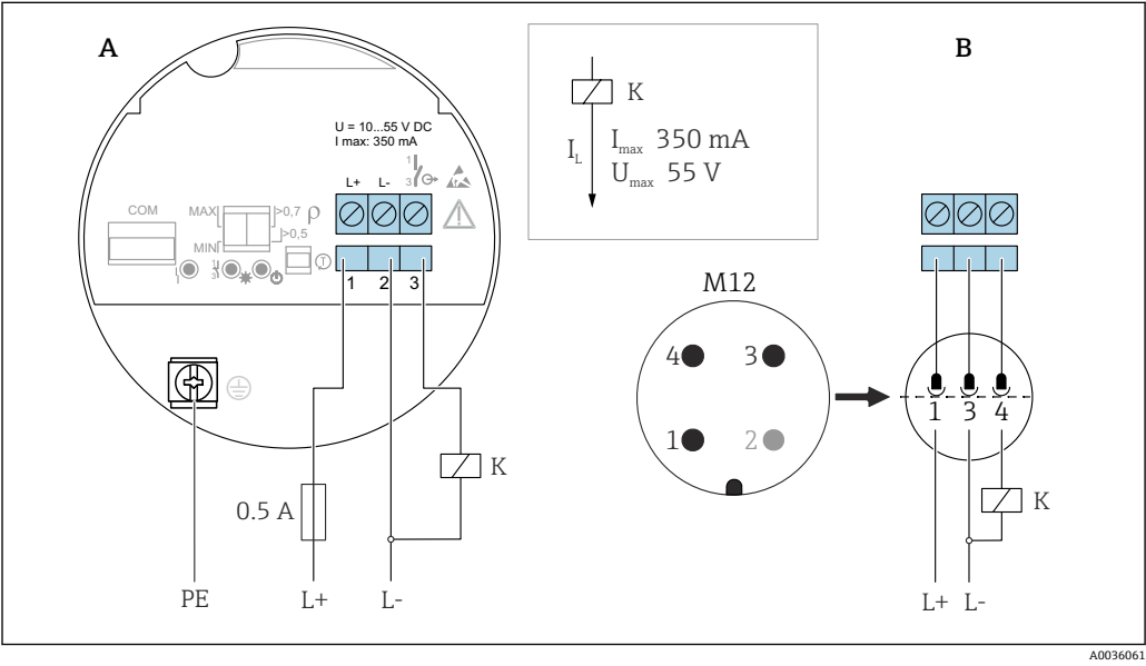
图 19 电子插件 FEL62: 三线制连接, 直流 DC-PNP 型
