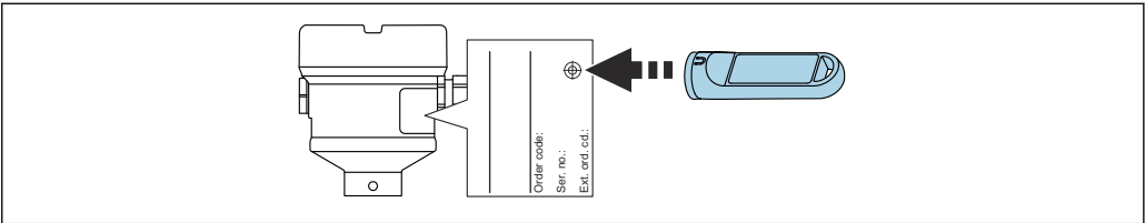
41 使用测试磁铁进行功能测试
