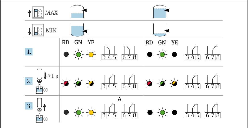
37 FEL64、FEL64DC 的继电器响应和故障报警信号
