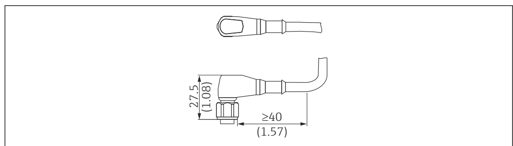
图 46 M12 插头，IP69 防护等级。测量单位 mm (in)
