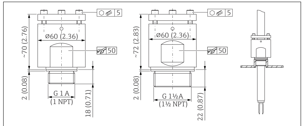
📖 51 高压滑动套管。测量单位 mm (in)
