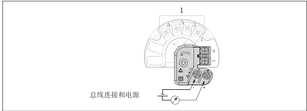
图 9 浪涌保护器的电气连接示意图
