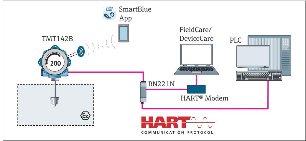
图 12 通过 HART®和 Bluetooth®蓝牙通信操作变送器
