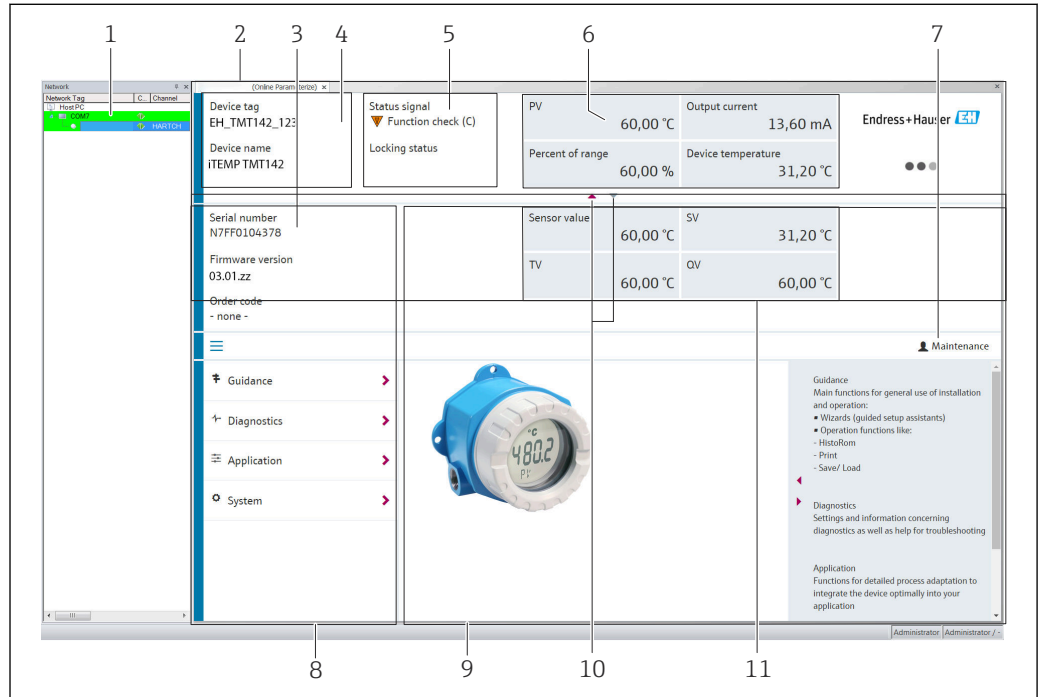
图 15 FieldCare 用户界面，显示设备信息
