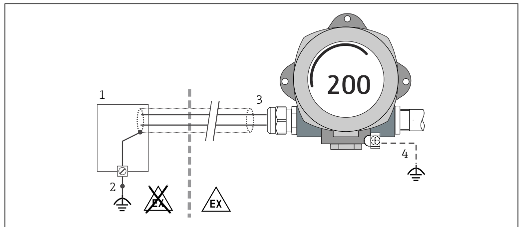
图 8 HART®通信电缆的单端屏蔽和接地连接
