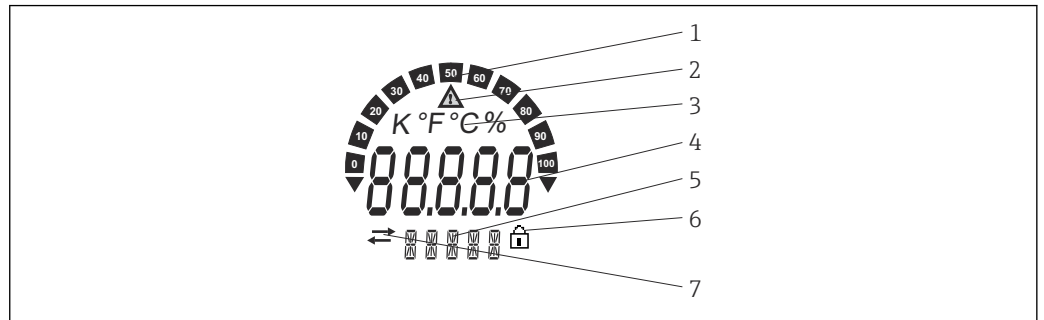
图 14 现场型变送器的液晶显示屏（背光显示，可插拔，每次旋转 90°）
