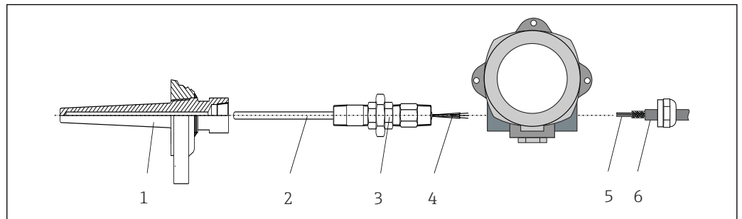
图 1 现场型变送器直接安装在传感器上
