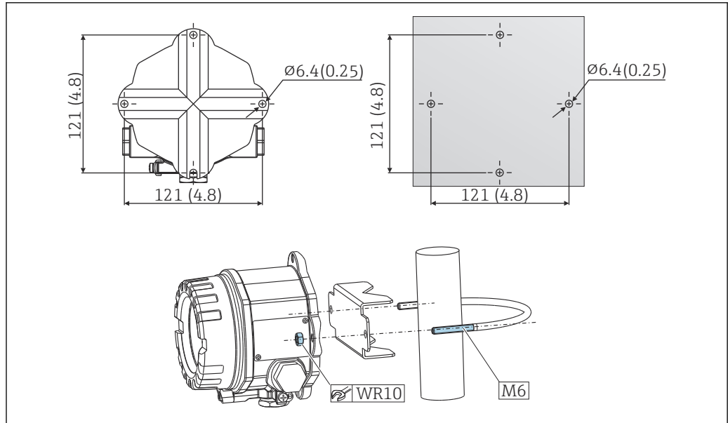
图 2 直接在墙壁上安装现场型变压器，或使用 2"管装架（316L）安装，参见“附件”章节；单位：mm (in)
