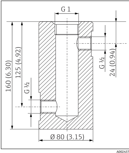
图 6 单位: mm (inch)
