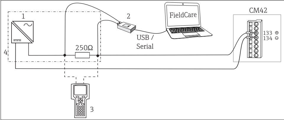
图 20: 未集成 PLC 的 HART 系统
