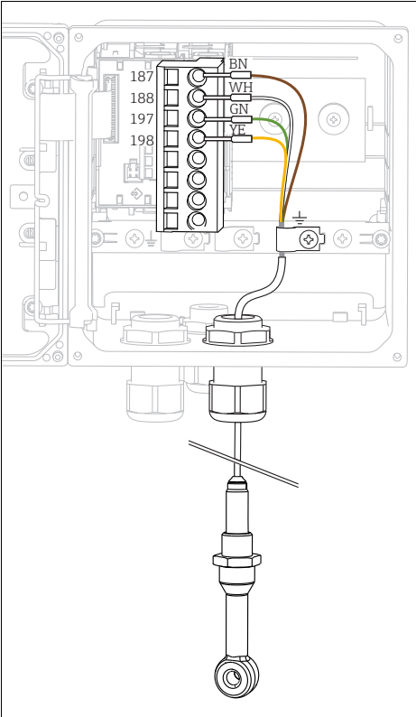
18: 设备内部视图
