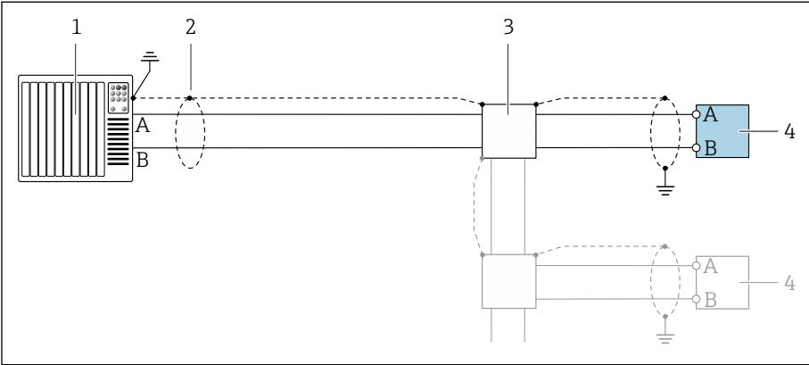
7 接线示例，Modbus RS485，非防爆区和防爆区（Zone 2；Cl. I, Div. 2）
