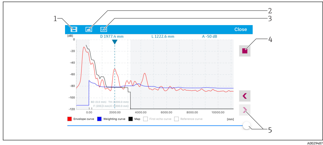
图 36 在 SmartBlue 中显示包络线; IoS 视图
