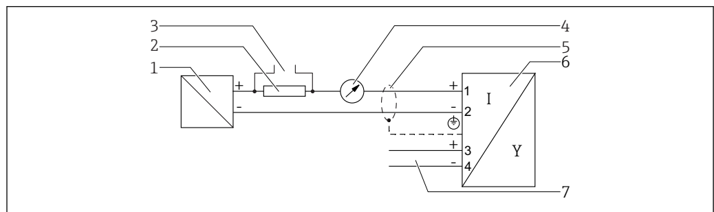
图 12 接线图：两线制；4...20 mA HART，开关量输出
