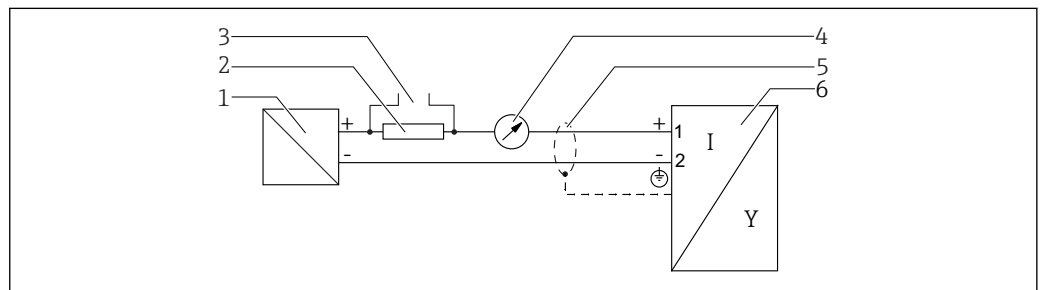
图 10 接线图: 两线制; 4...20 mA HART
