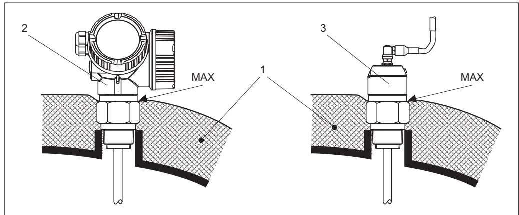
图 6 带螺纹过程连接的 FMP50
