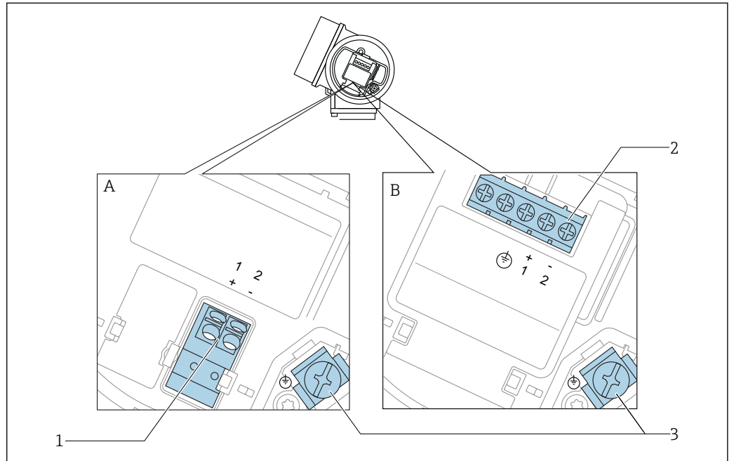
图 9 接线端子分配: 两线制; 4...20 mA HART
