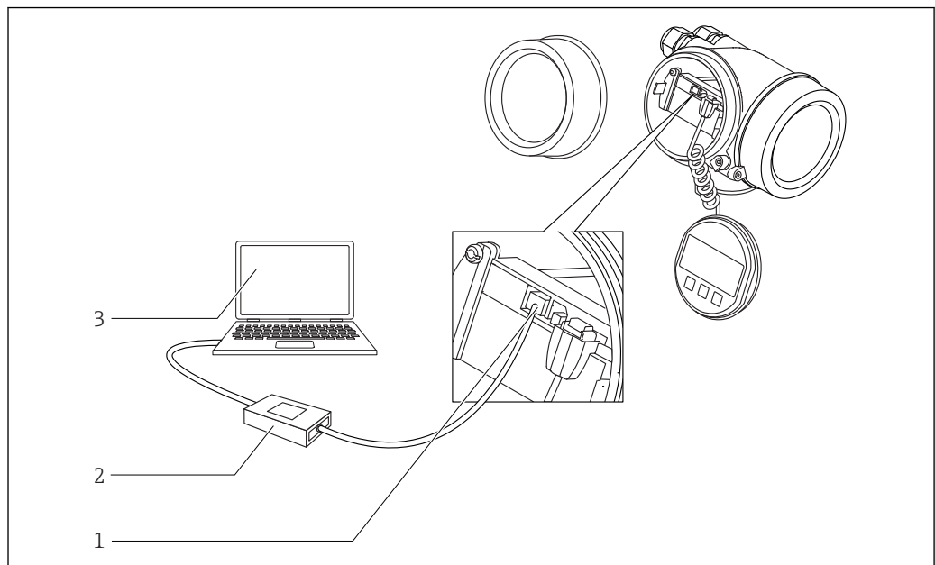
图 27 DeviceCare/FieldCare, 使用服务接口 (CDI)
