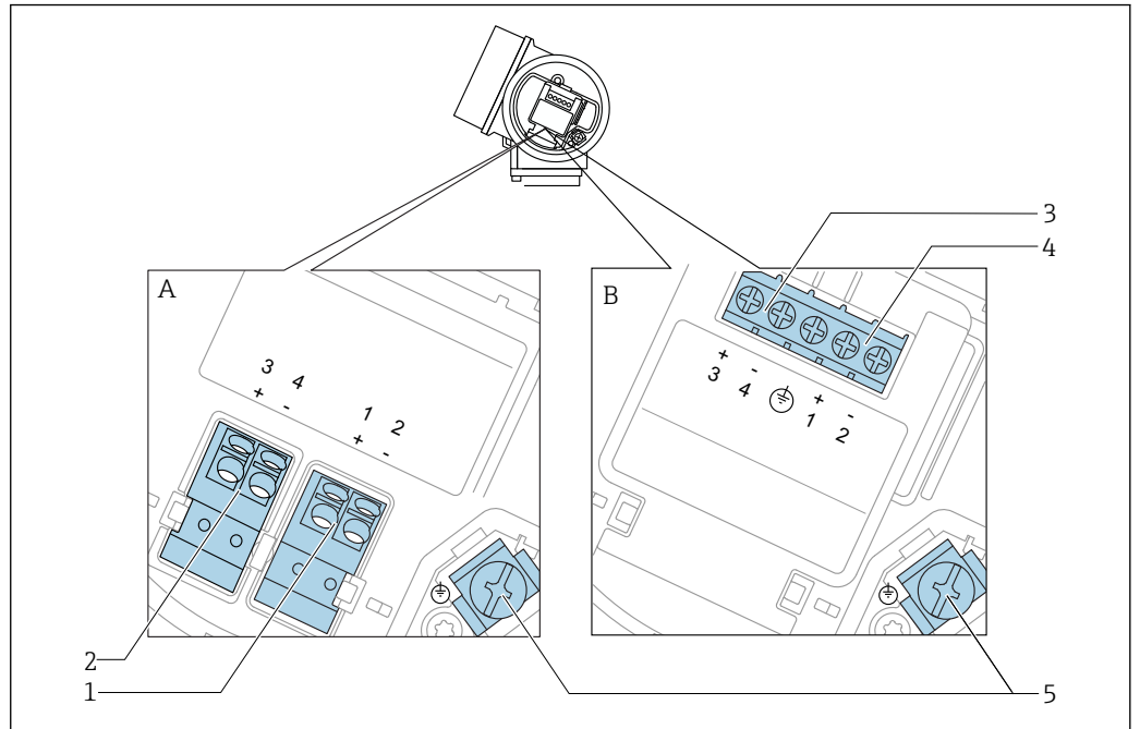
图 13 接线端子分配: 两线制; 4...20 mA HART, 4...20 mA
