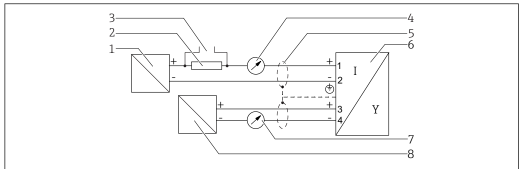
图 14 接线图: 两线制; 4...20 mA HART, 4...20 mA
